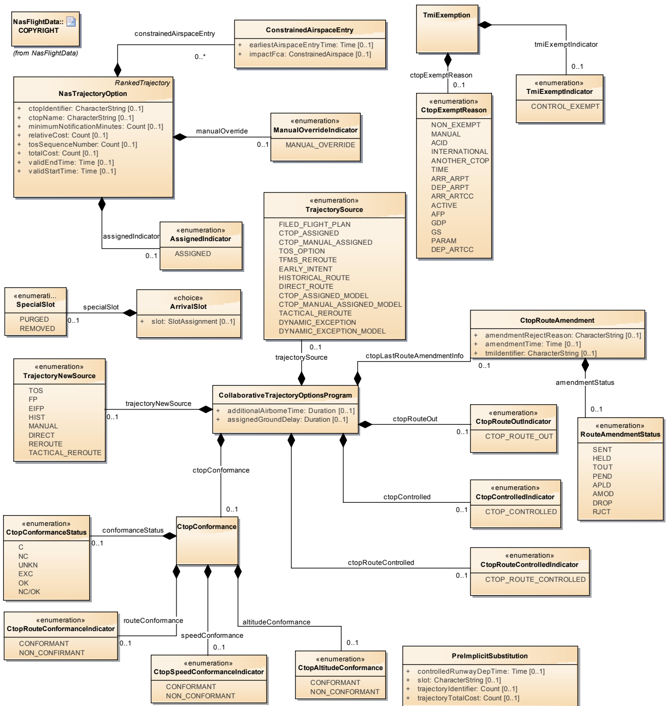
Figure 20: NasTrajectoryOptions
